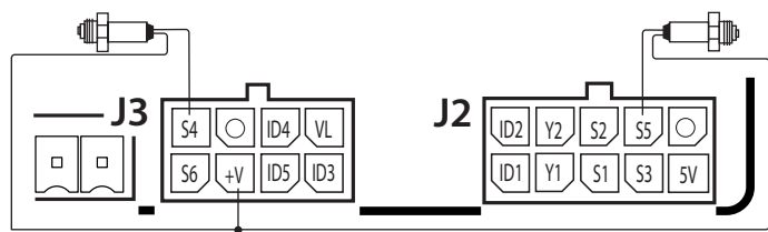
Цифровые входы/датчики 4-20 мА
