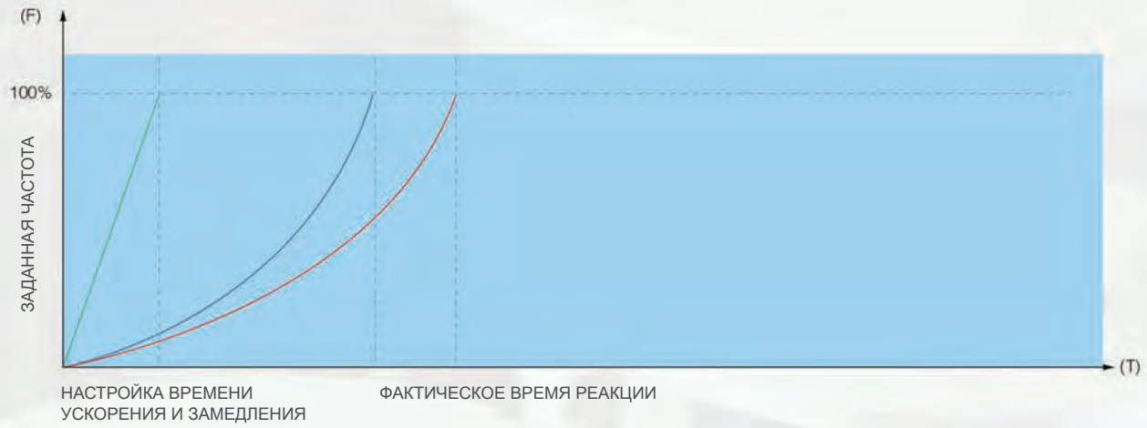
сравнение динамических характеристик в различных режимах управления
