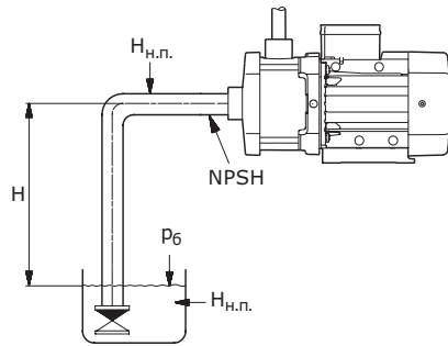
Рис. 9 Минимальное давление на входе
