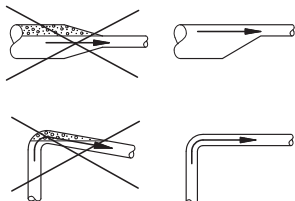
Рис. 4 Трубопровод
