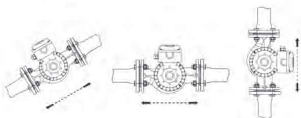
Рис. 59 Варианты монтажа
