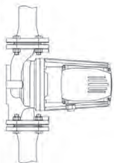
Рис. 16 Положение вала электродвигателя
