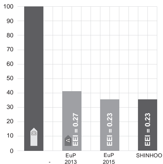
Рис. 2 Индекс энергопотребления
