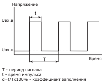
Рис. 16 Характеристики ШИМ-сигнала
