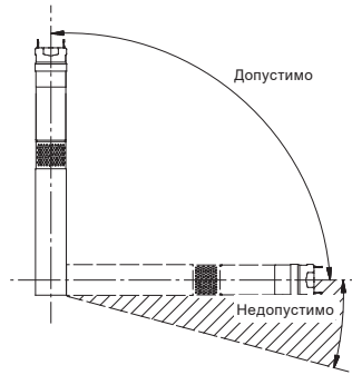
Рис. 11 Правильное монтажное положение SQ, SQE, SQF
