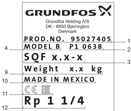
Рис. 7 Фирменная табличка скважинных насосов SQF (Helical)
