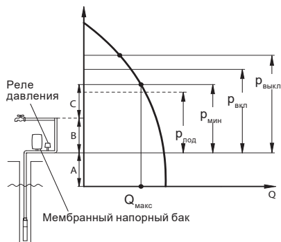
Рис. 21 Выбор давления в системе
