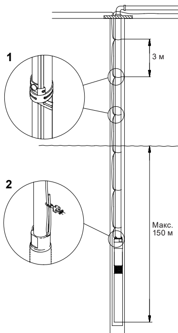
Рис. 19 Подсоединение к трубопроводу
