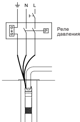
Рис. 20 Реле давления
