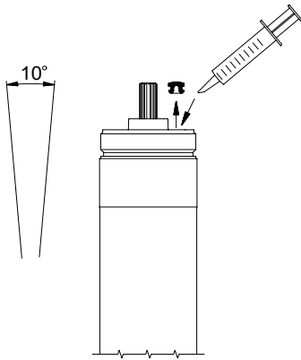
Рис. 10 Доливка жидкости в электродвигатель
