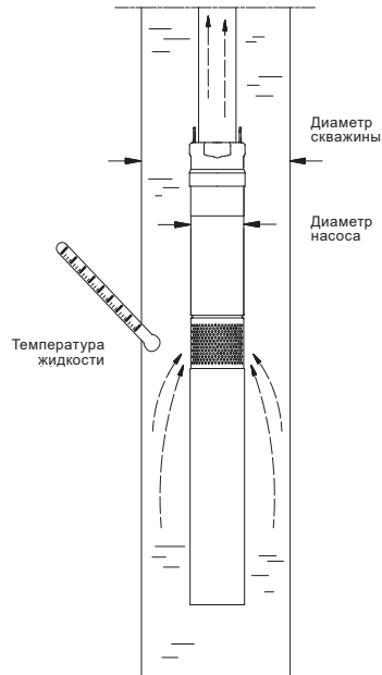
Рис. 12 Насос SQ/SQE, установленный в буровой скважине
