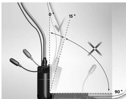
Рис. 8 Положение насосов/установок SB, SBA
