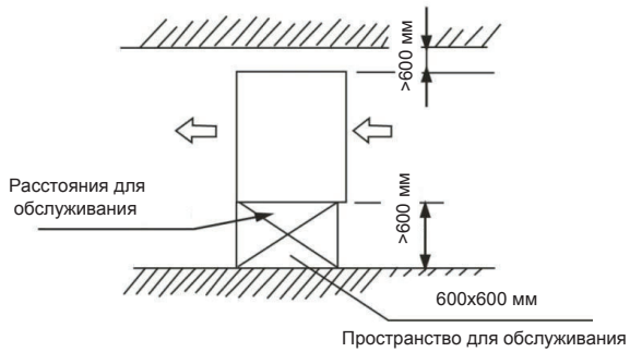
Вид сверху
