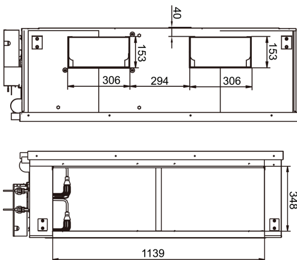
Вид сверху
