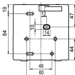
Вид сзади
