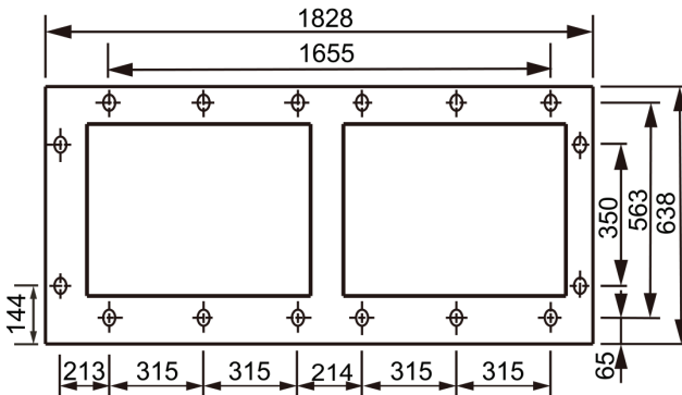
Вид сзади
