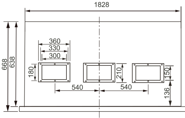
Вид спереди
