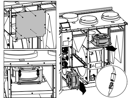
Рис. 3 Приточный и вытяжной вентиляторы
