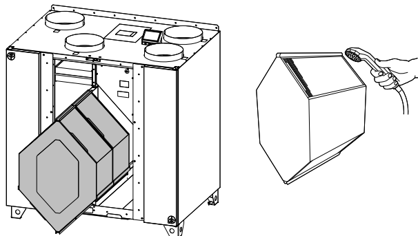
Рис. 5 Снятие и чистка теплообменника
