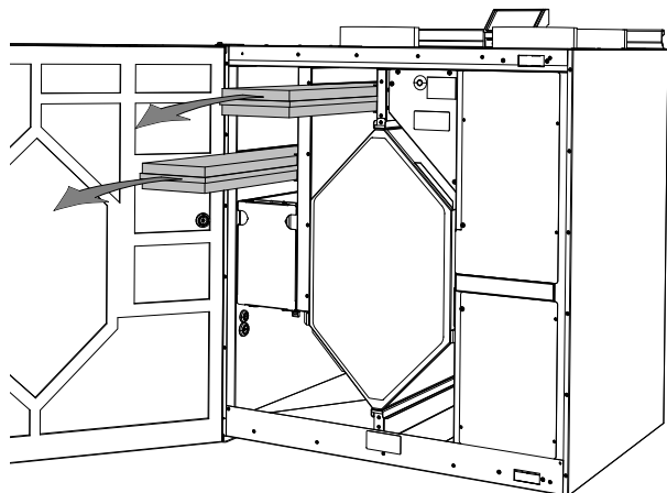
Рис. 3 Замена фильтров
