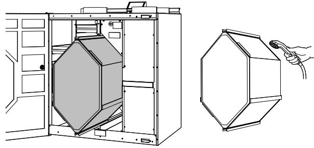
Рис. 4 теплообменник
