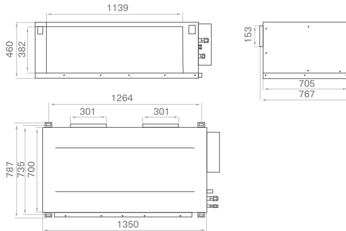
SAD80D3-A, SAD100D3-A
