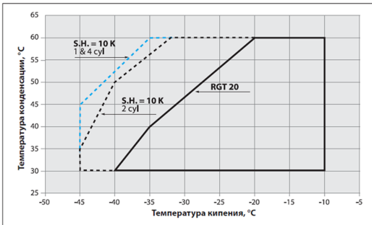
Область эксплуатации компрессоров NTZ с хладагентом R404A/R507A S.H. перегрев, 1&amp;4 cyl- 1 и 4 цилиндры компрессоры, 2 cyl – 2-цилиндровые компрессоры, RGT20 – температура всасываемого газа.
