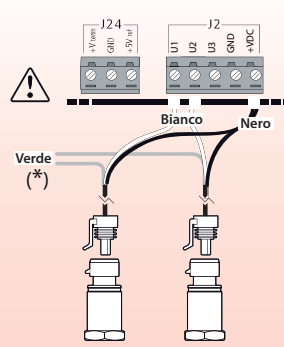
Sonda 4-20 mA:
