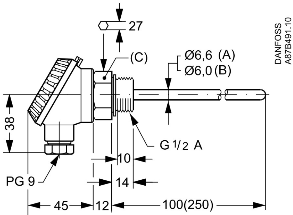
Габаритные размеры датчика температуры типа ESMU.
